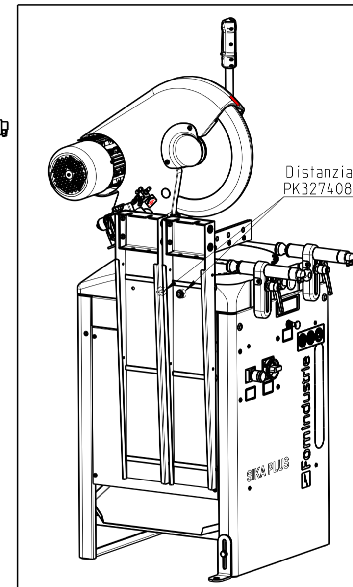
Montaggio reggi profilo laterale per il trasporto Side profile support assembly for transport
